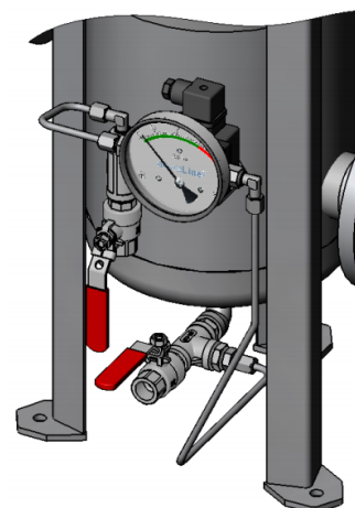
DP-Indikator och anslutningsrör
