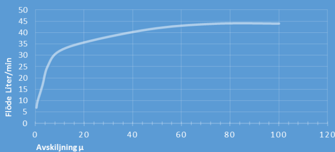
MAX FLÖDE PER 10" VID TRYCKFALL 0,15 BAR
